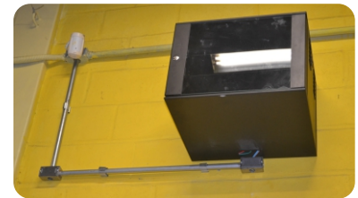
Reforma lógica e elétrica Hipercard - Sam's Club - Santa Rita/PB
