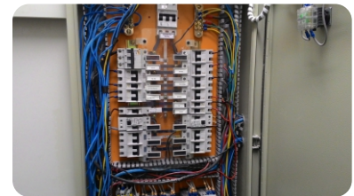
Manutenção em Quadros elétricos Unimed - Recife/PE
